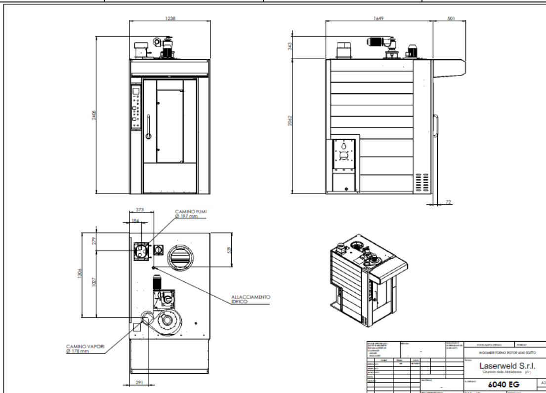
Dis. 5.1 Forno Rotor 6040/5070 innesti superiori
